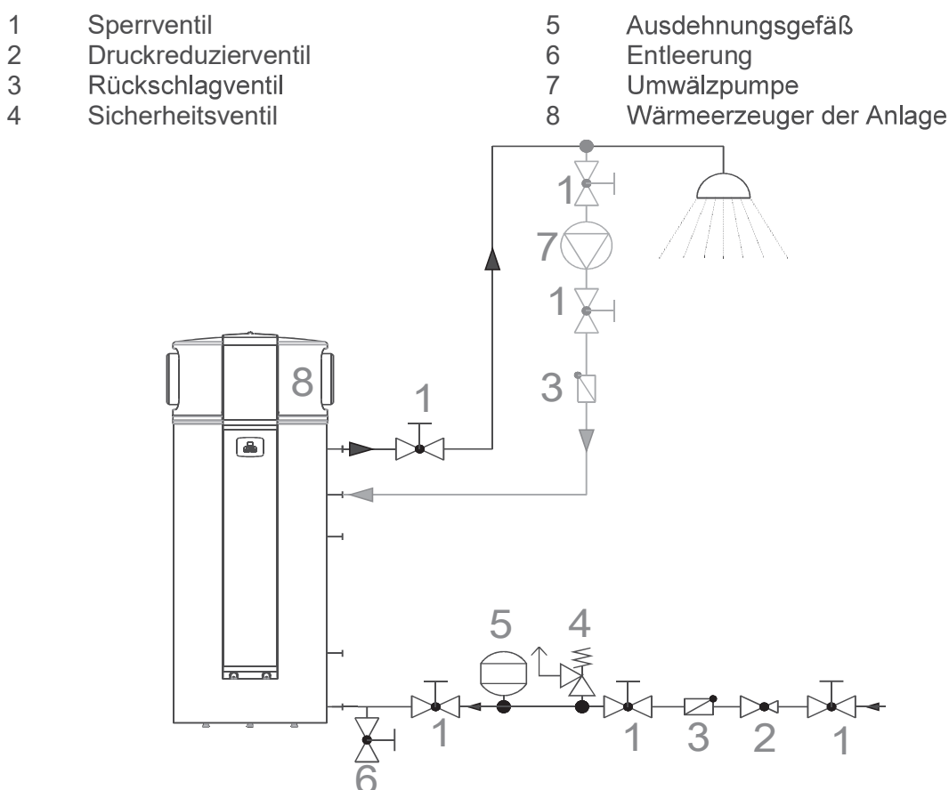
Abbildung 7: Anschluss ans Wasserversorgungsnetzwerk
